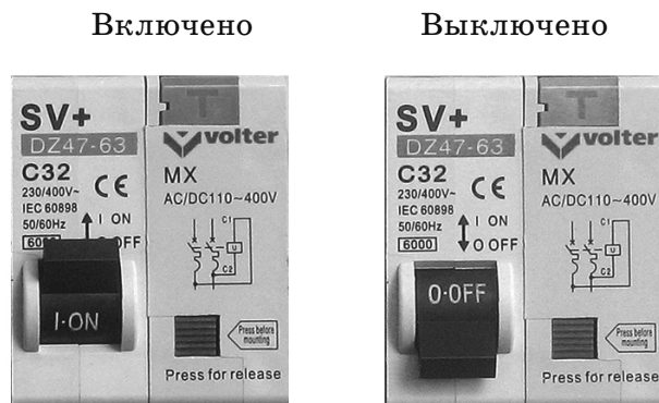
Рис.3. Положение автоматического выключателя
